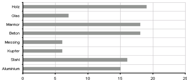
Durchschnittliche Scherfestigkeit bei Überlagerung (N/mm 2 ) unterschiedlicher Materialien
