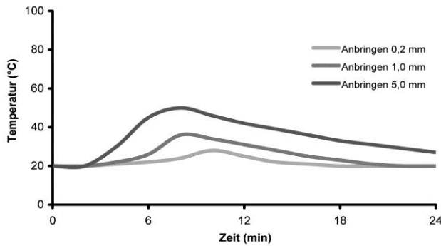
Temperaturkurve der Reaktion für Anwendungen bei 20°C
