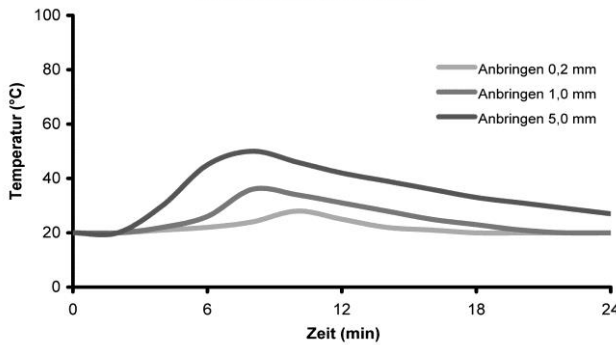
Temperaturkurve der Reaktion für Anwendungen bei 20°C
