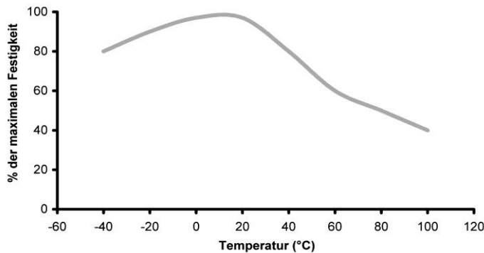
Durchschnittliche Scherfestigkeit bei Überlagerung bezogen auf eine Aushärtung von 48 H bei 20°C
