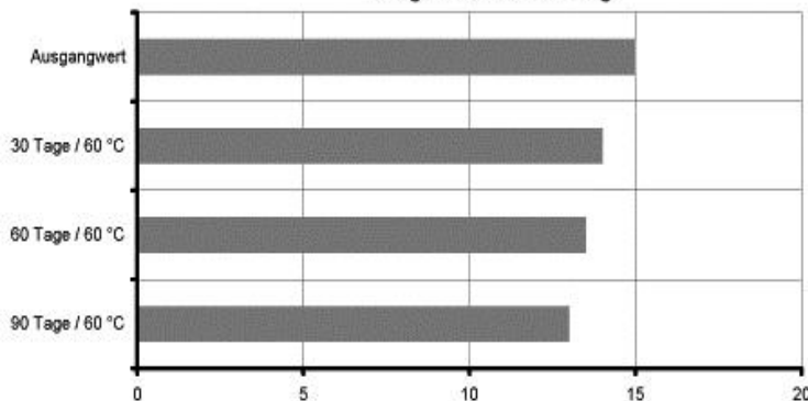
Durchschnittliche Scherfestigkeit bei Überlagerung (N/mm 2 ) bezogen auf Wärmealterung
